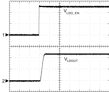
LDO Enable
